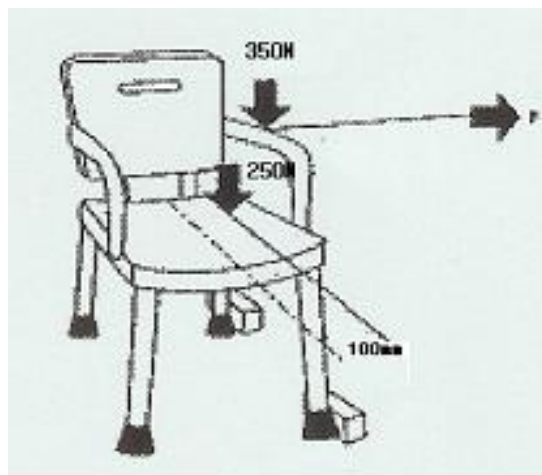
그림 3 — 팔걸이부착 측방안정성시험
