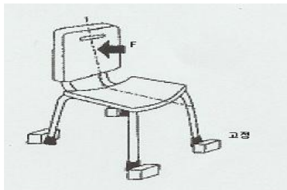
그림 13 — 등받이 내구성시험
