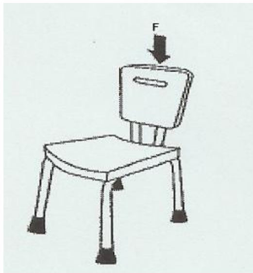
그림 7 — 등받이 수직안정성시험
