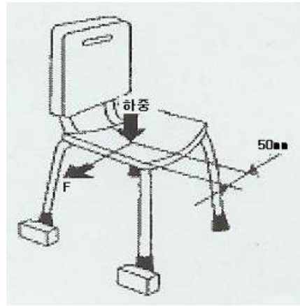
그림 2 — 팔걸이 없는 제품 측방안정성시험
