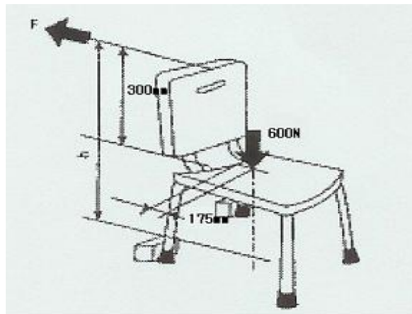
그림 5 — 등받이 후방안정성시험
