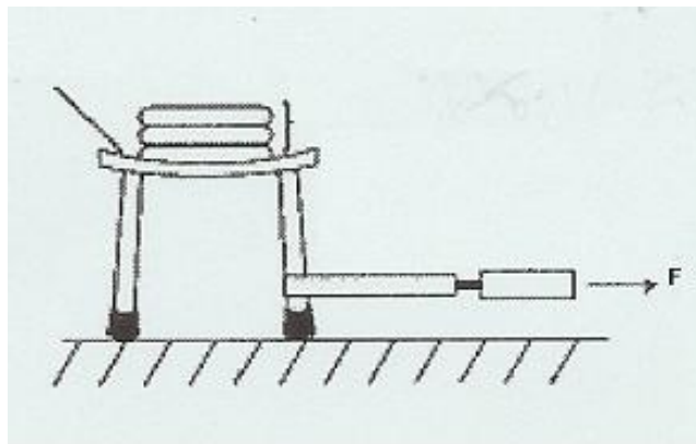
그림 15 — 미끄럼저항시험
