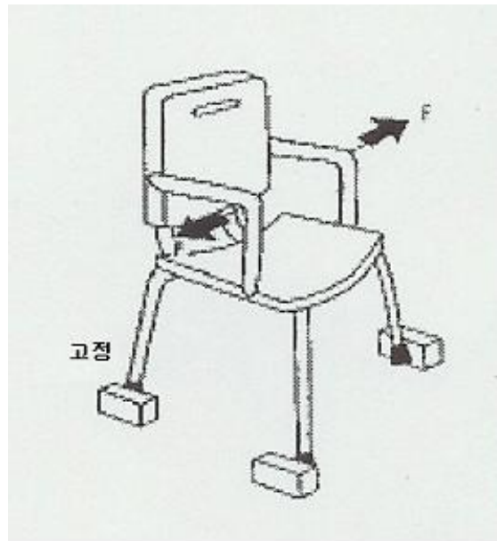
그림 10 — 팔걸이 정적강도시험
