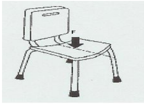
그림 12 — 좌면 내구성시험
